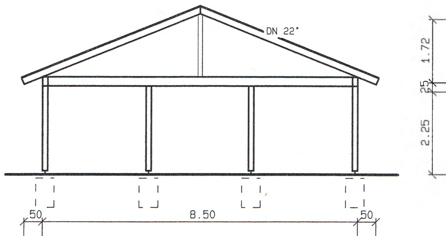
Ansicht Giebel
